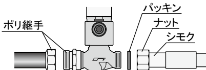
(例 1次側：ポリエチレン管接続、2次側：鋼管接続)
