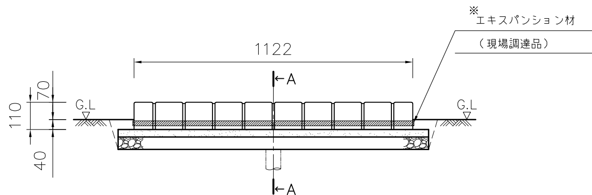
立面図
