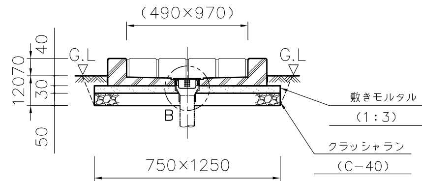
A-A断面図
