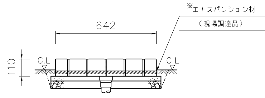
A-A断面図
