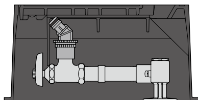
接続継手 (R1/2)
